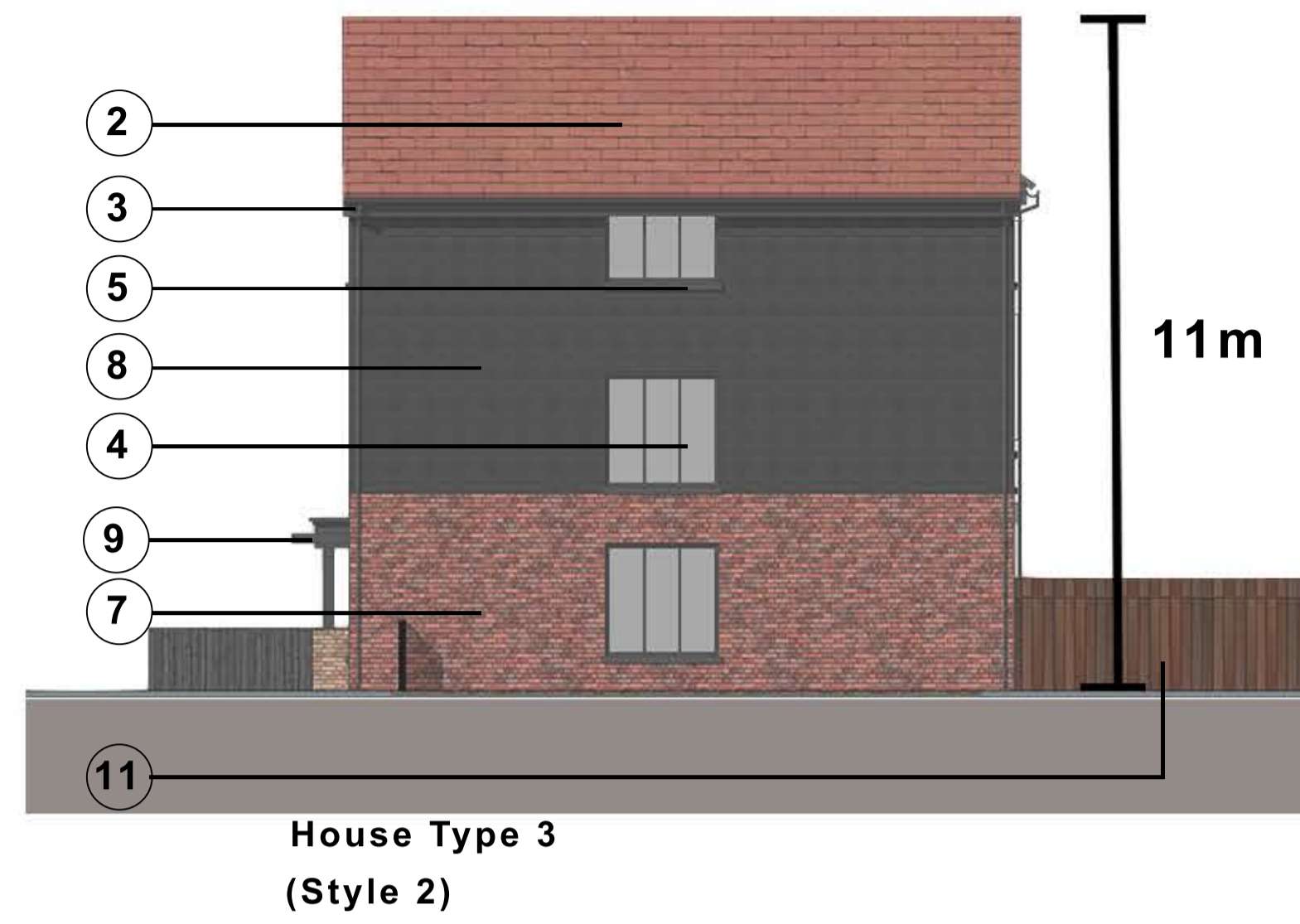
ELEVATION 2
